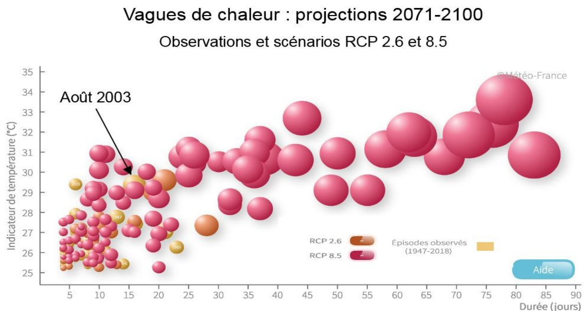
Figure 1 : vagues de chaleur observées et simulées en l'absence de politique climatique (i.e. scénario RCP 1 8,5) – source : Météo France.
